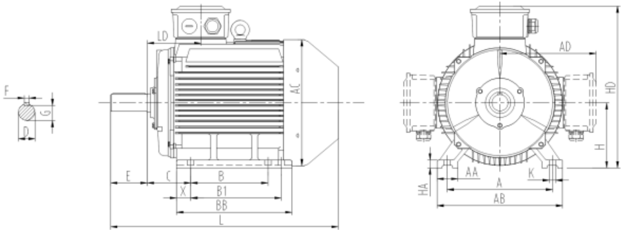
机械尺寸数据(Outline&Installation Dimensions) B3
