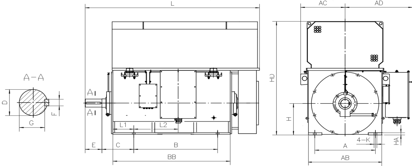
• 安装尺寸表MOUNTING DIMENSIONS FOR INSTALLATION
