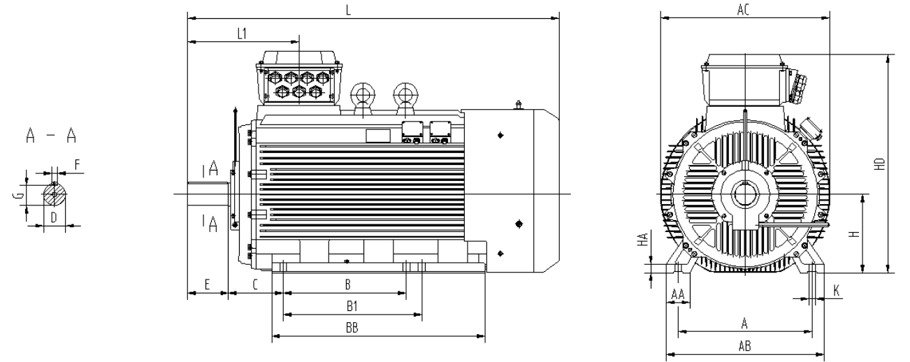
机械尺寸数据 ( Outline&Installation Dimensions) B3
