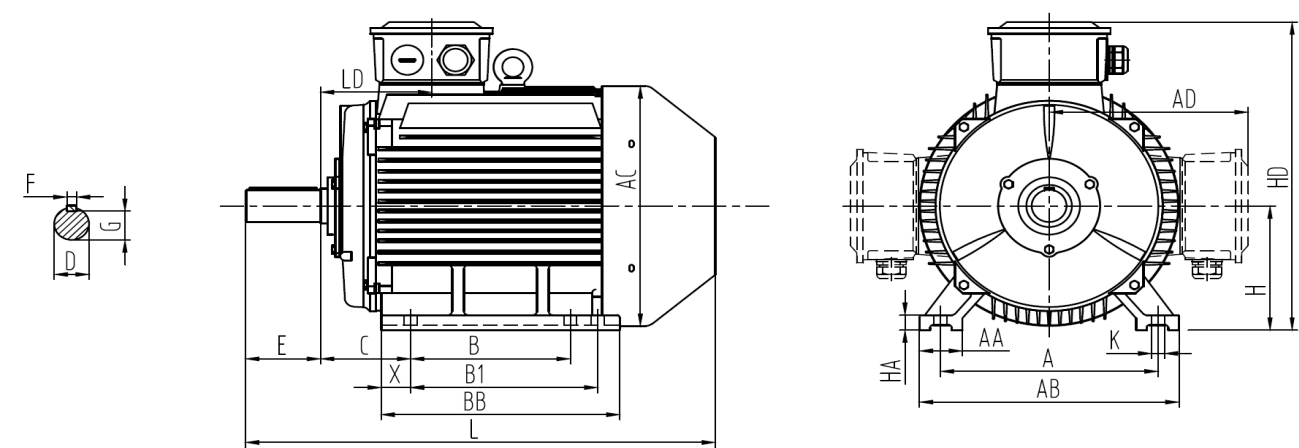
机械尺寸数据 (OMT4) Outline&Installation Dimensions (OMT4) B3
