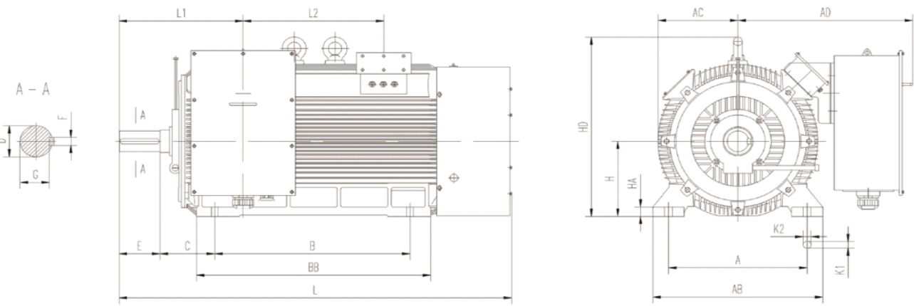
机械尺寸数据 (Outline&Installation Dimensions)
