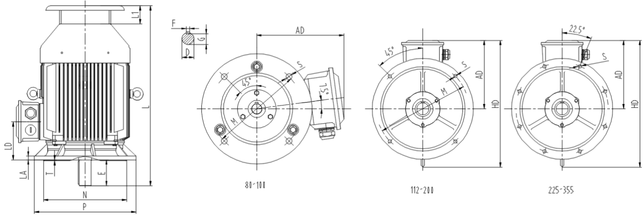
机械尺寸数据 (Outline&Installation Dimensions) V1
