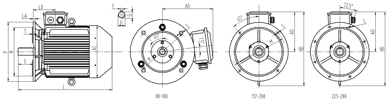
机械尺寸数据 (OMT4) Outline&Installation Dimensions (OMT4) B5
