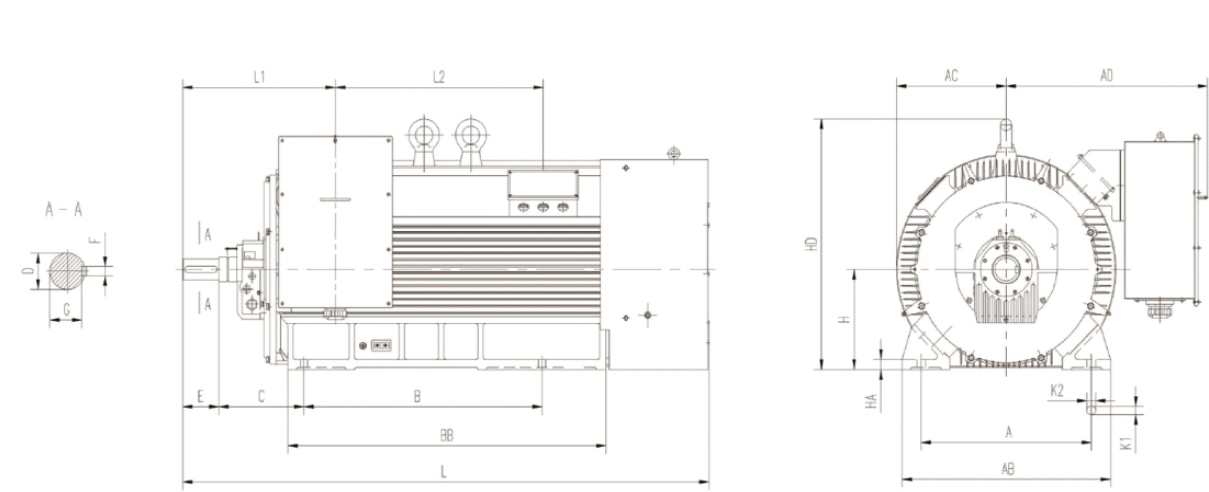
机械尺寸数据 (Outline&Installation Dimensions)
