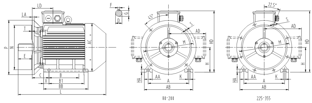
机械尺寸数据 (Outline&Installation Dimensions) B35
